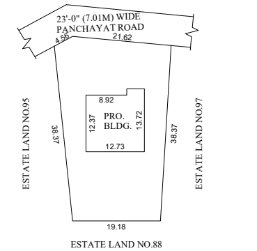
SITE PLAN (SCALE 1:400)
