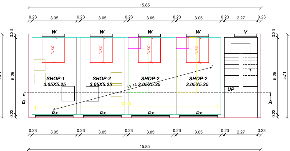
DOOR PLAN
