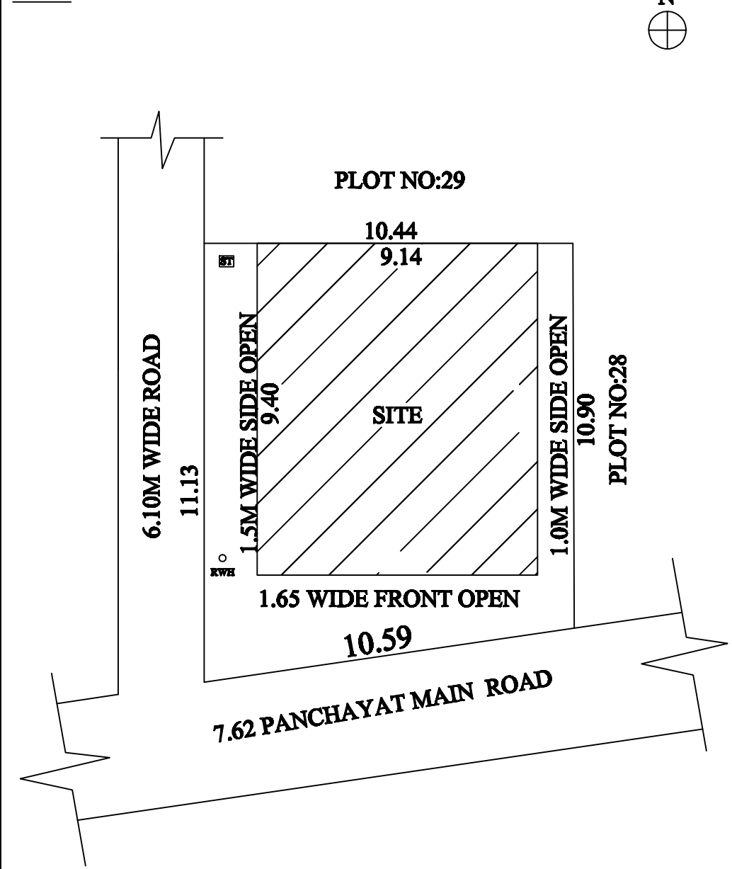
SITE PLAN: 1:200
