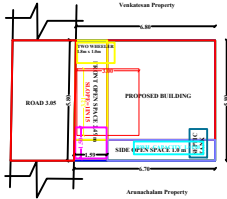
SITE PLAN: SCALE 1:100
