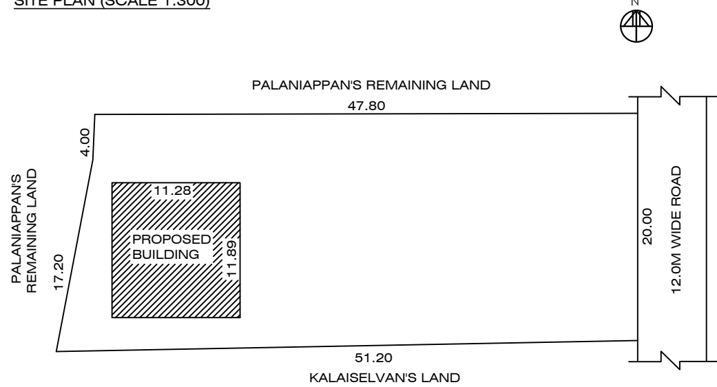
SITE PLAN (SCALE 1:300)
