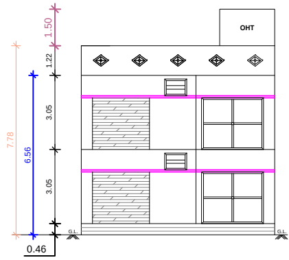
ELEVATION-A
