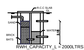
LONGITUDINAL SECTION
