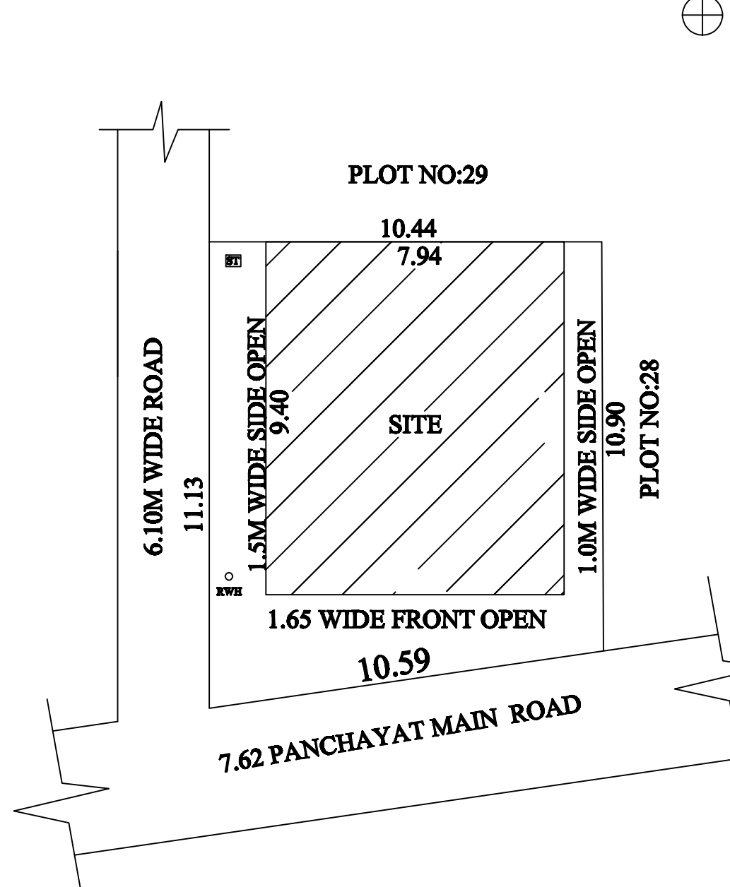
SITE PLAN: 1:200
