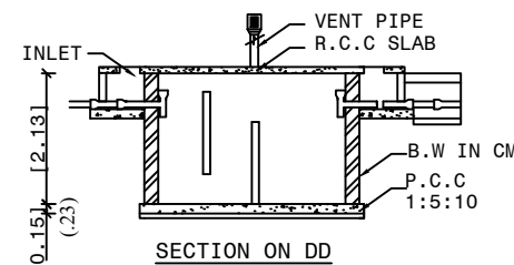
SECTION ON DD
