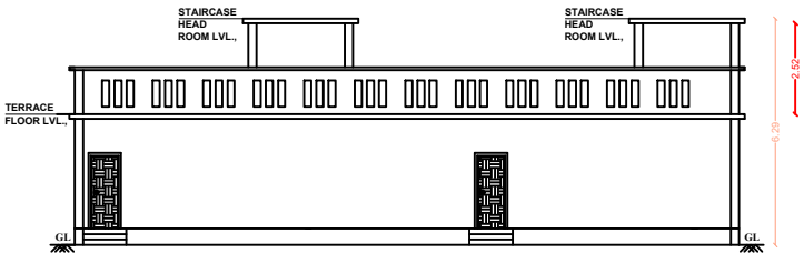
ELEVATION
