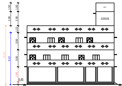
ELEVATION-A
