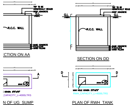
PLAN OF R.W.H. TANK
