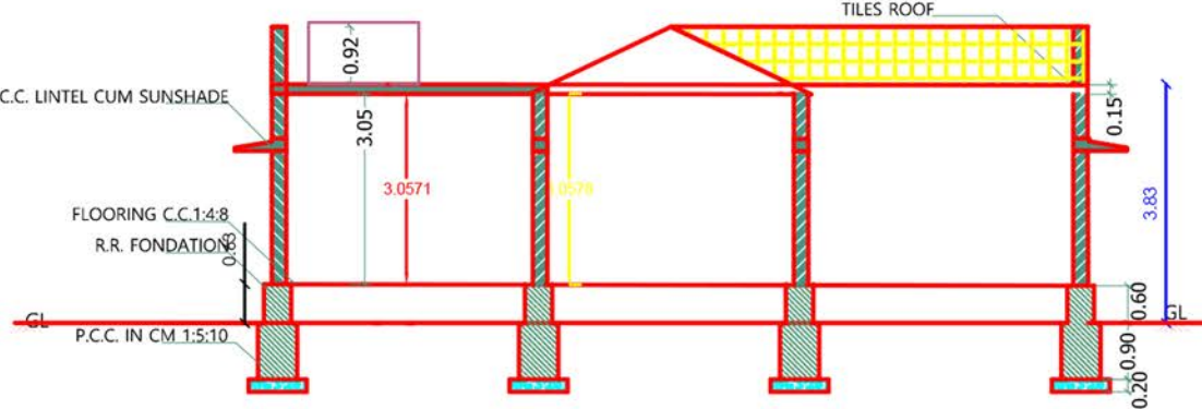
SECTIONN A-A
