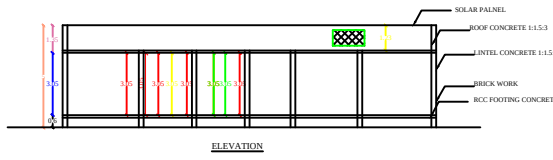
ELEVATION
