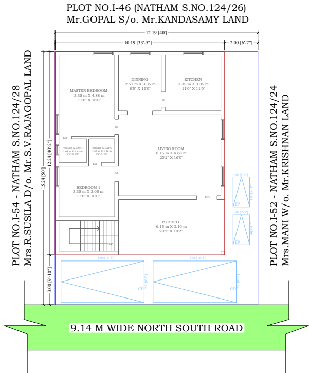
SITE PLAN(SCALE -1:250)
