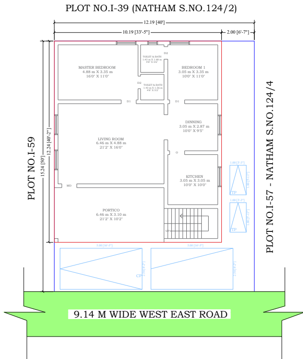
SITE PLAN(SCALE - 1:250)
