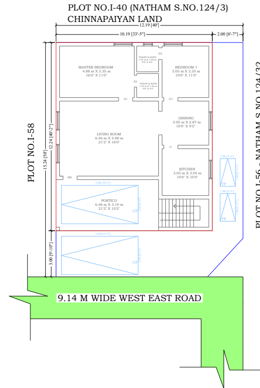
SITE PLAN(SCALE - 1:250)
