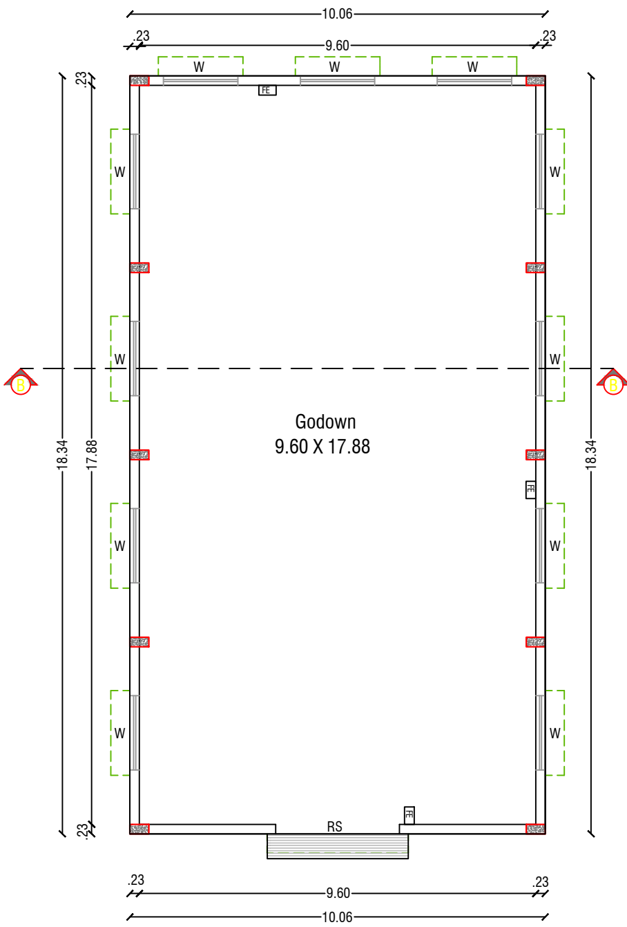
GODOWN PLAN
