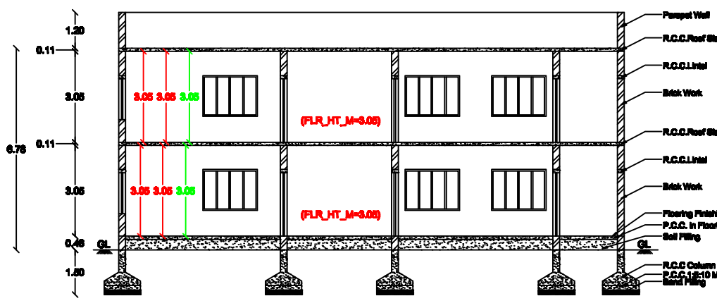
SECTION CH AA
