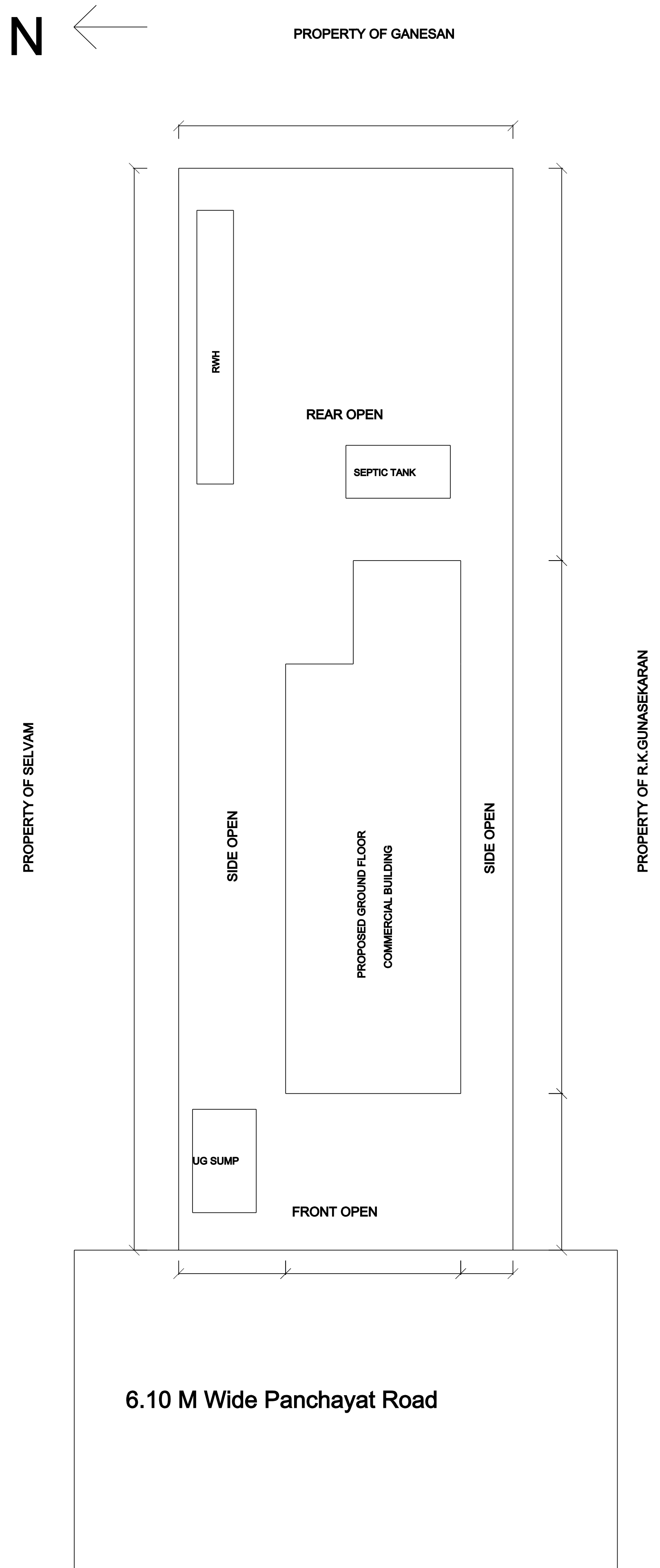
SITE PLAN 1:100
