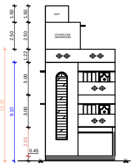
ELEVATION-A
