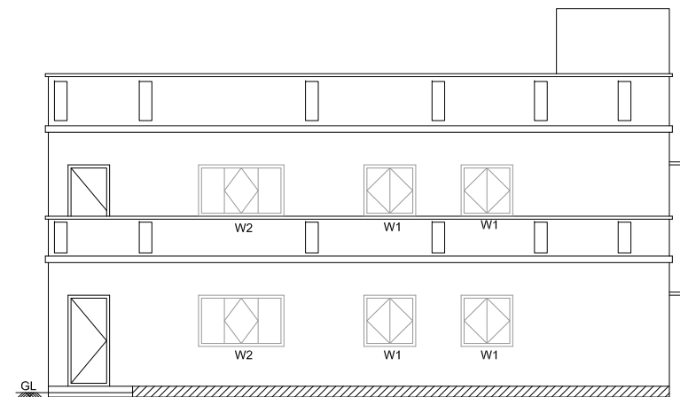
ELEVATION - A
