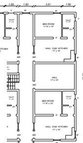
FLOOR PLAN 1,2
