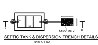
SCALE: 1:100
