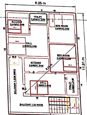
F.F. PLAN
