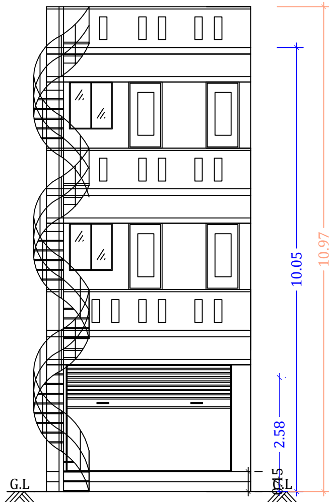
ELEVATION
