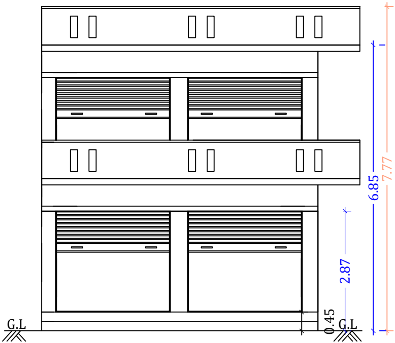
ELEVATION
