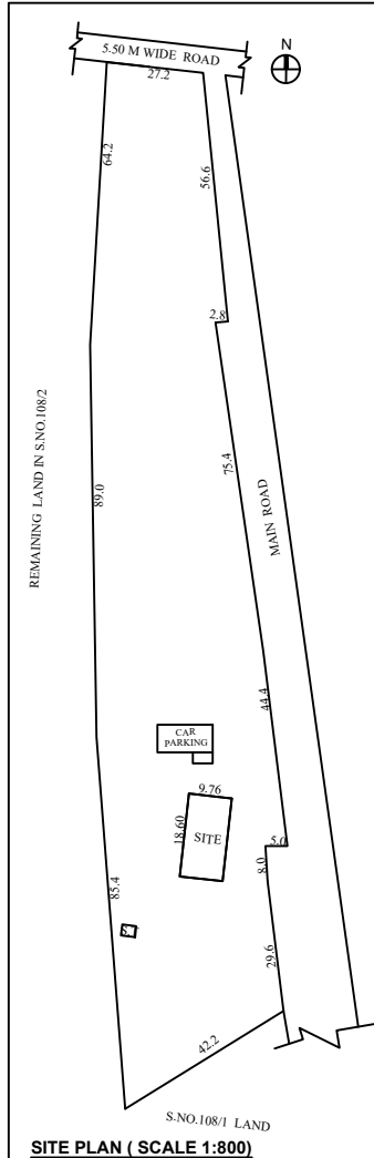
SITE PLAN ( SCALE 1:800)
