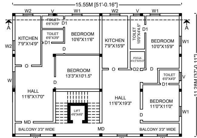
SECEND FLOOR PLAN
