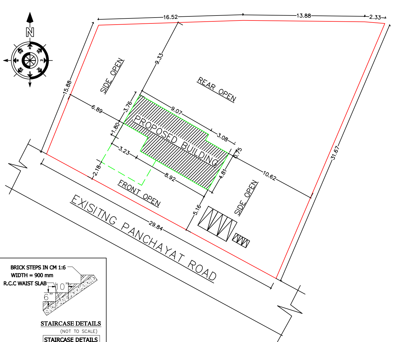
SITE PLAN (1 : 200)
