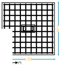
COLOUMN FOU
