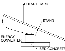
LONGITUDINAL SECTION
