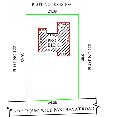
SITE PLAN (SCALE 1:400)
