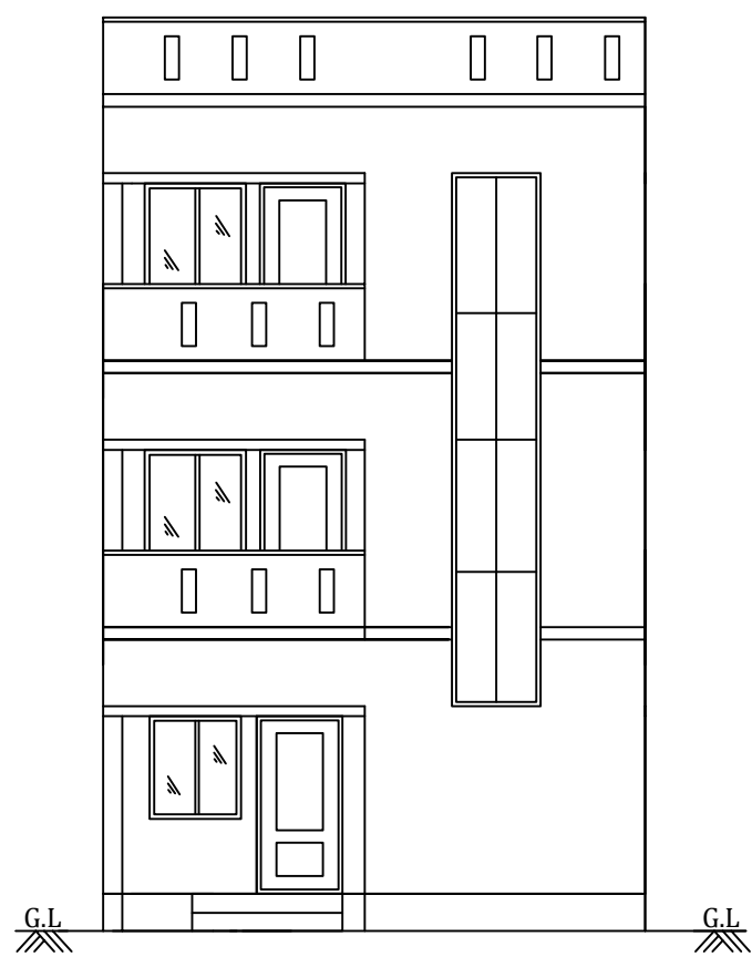
ELEVATION
