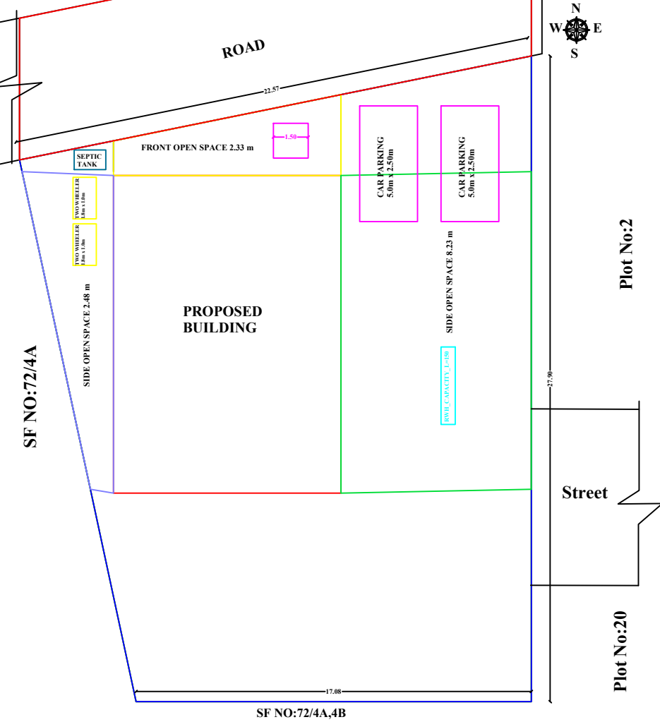
SITE PLAN 1:100 SCALE
