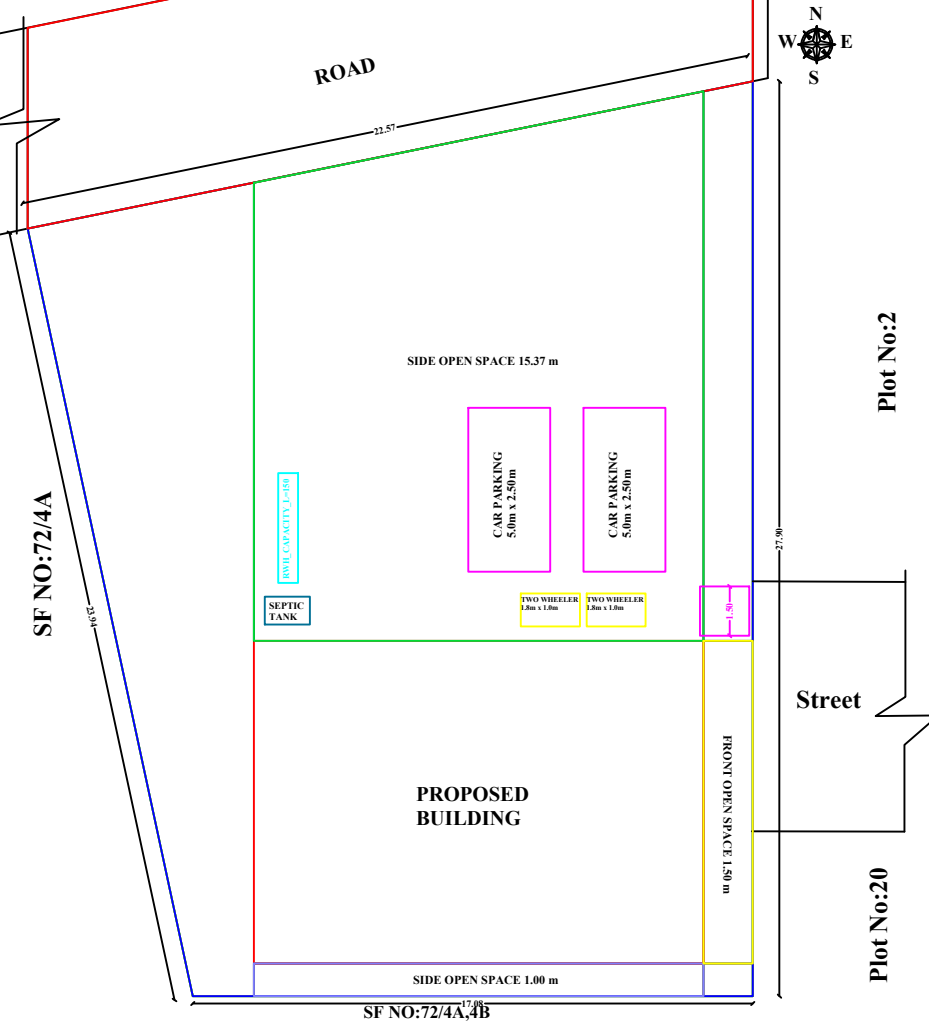
SITE PLAN 1:100 SCALE
