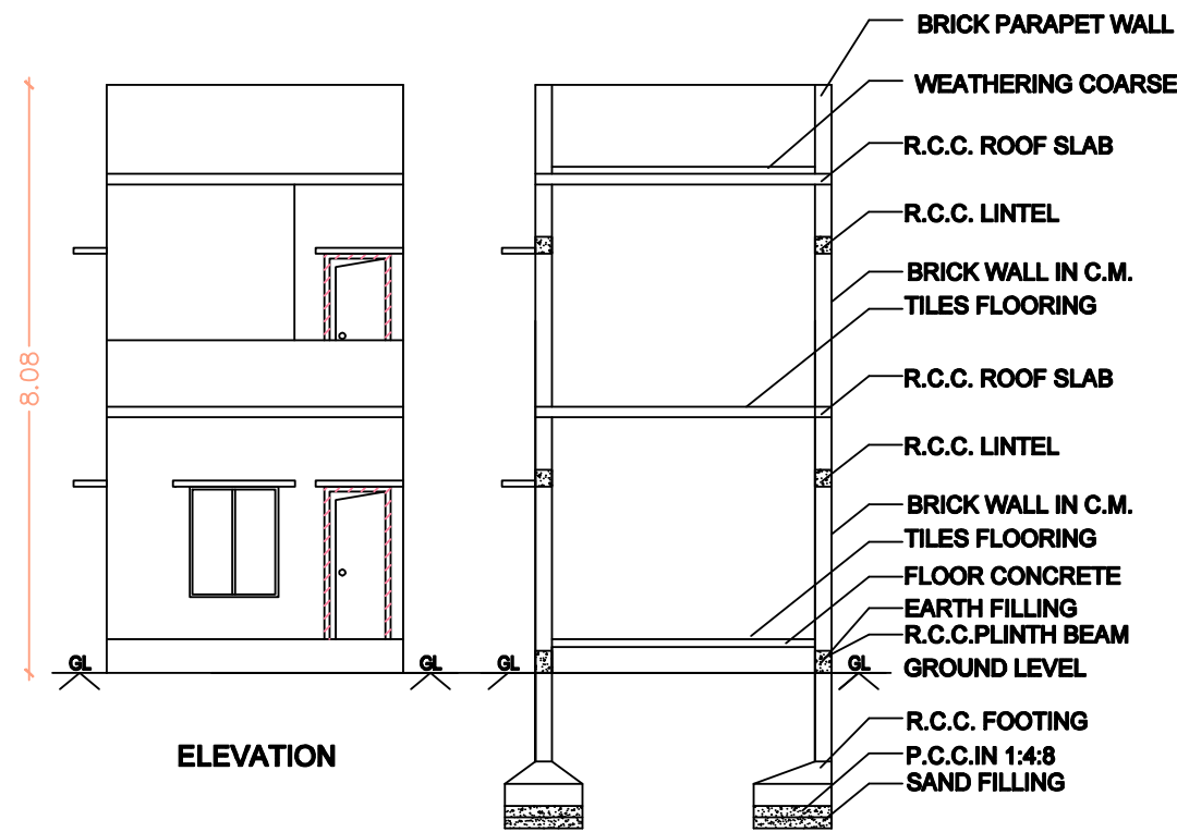
A-A SECTION
