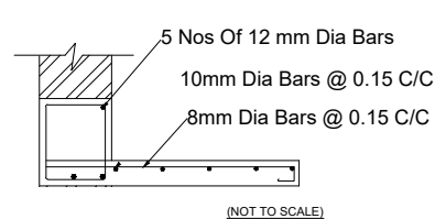
LINTEL CUM SUNSHADE DETAIL :
