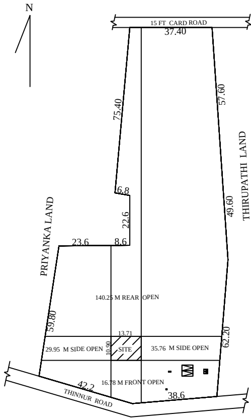
SITE PLAN NTS
