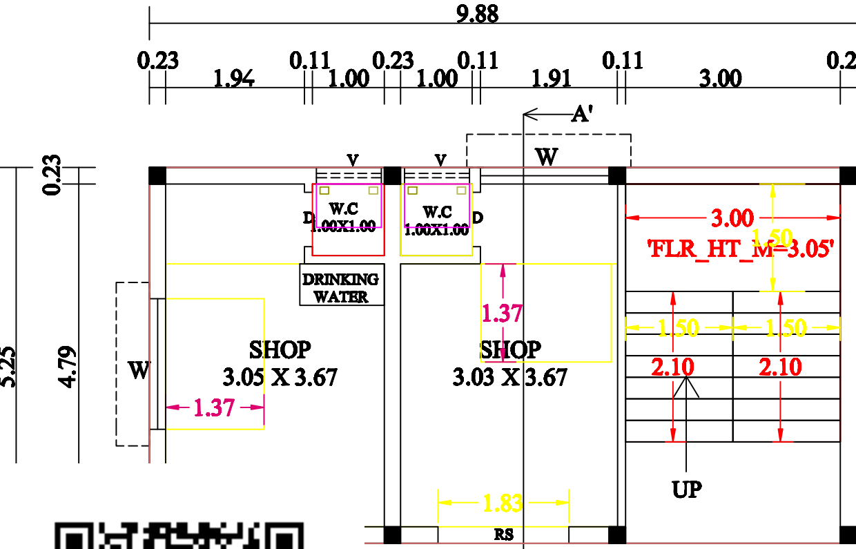
UND FLOOR PLAN
