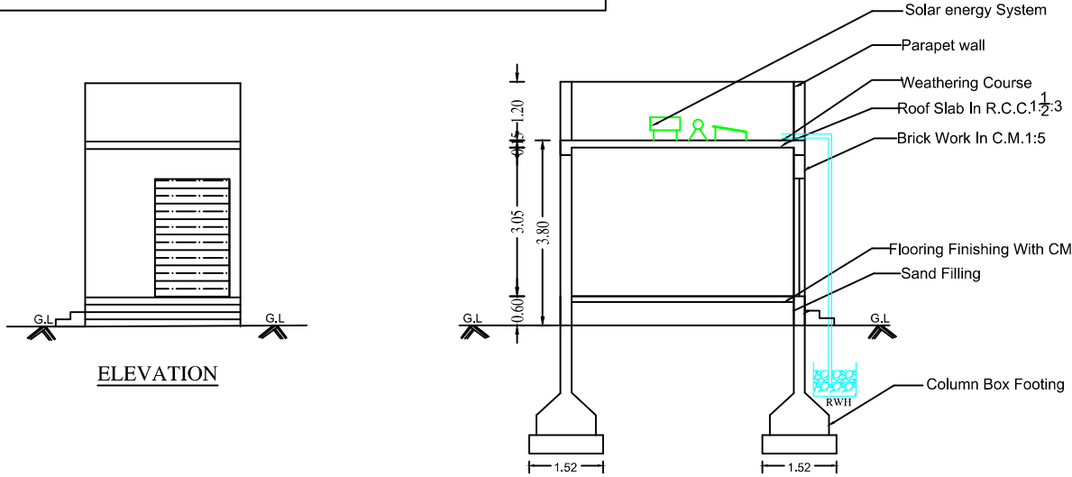
SECTION A-B
