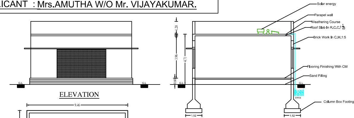
SECTION A-B
