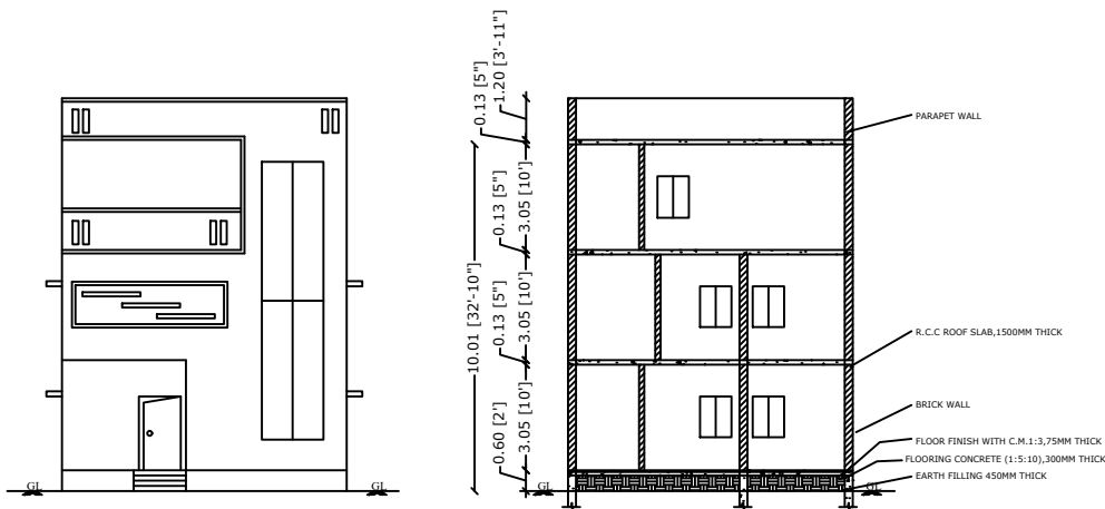
ELEVATION
