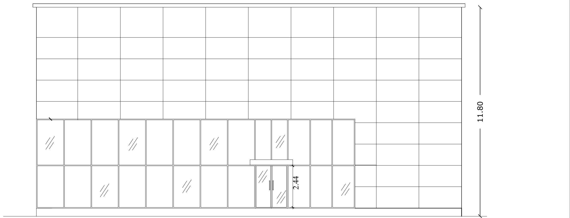
ELEVATION
