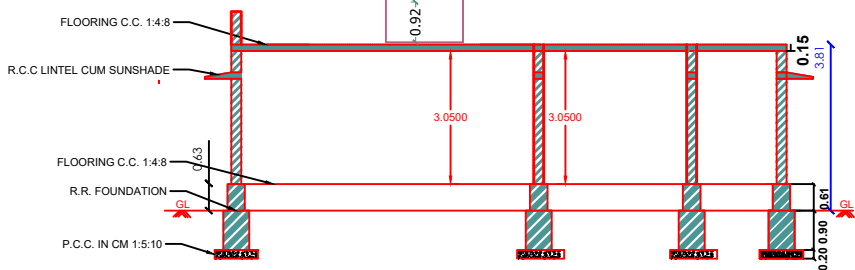
SECTIONN A-A
