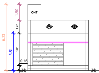
ELEVATION-A
