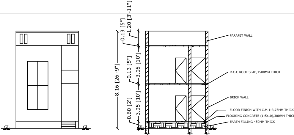
ELEVATION
