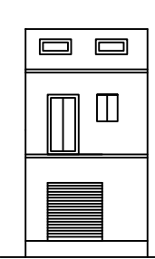
ELEVATION
