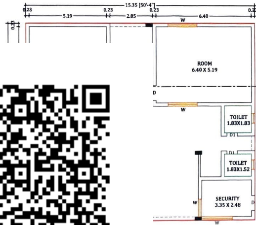
DOOR PLAN
