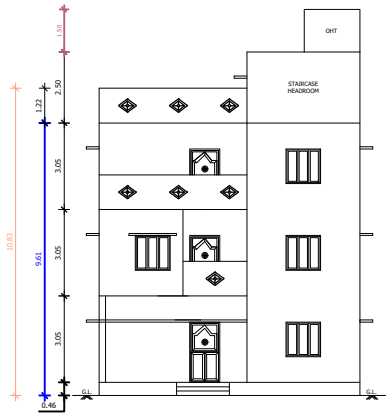
ELEVATION-A
