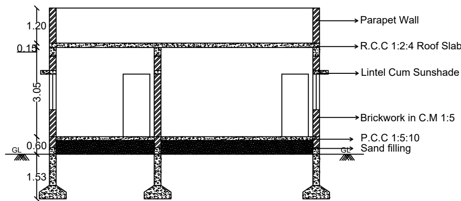
SECTION - AB
